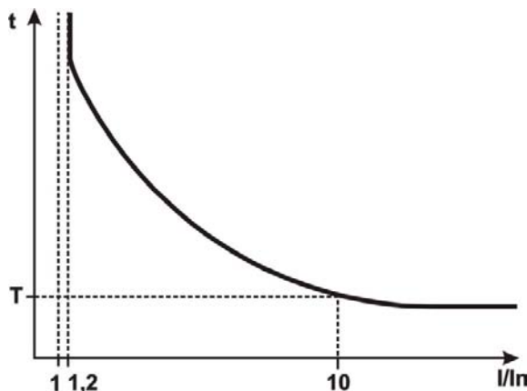
Рисунок 5 – Принцип работы защиты с зависимой выдержкой времени
