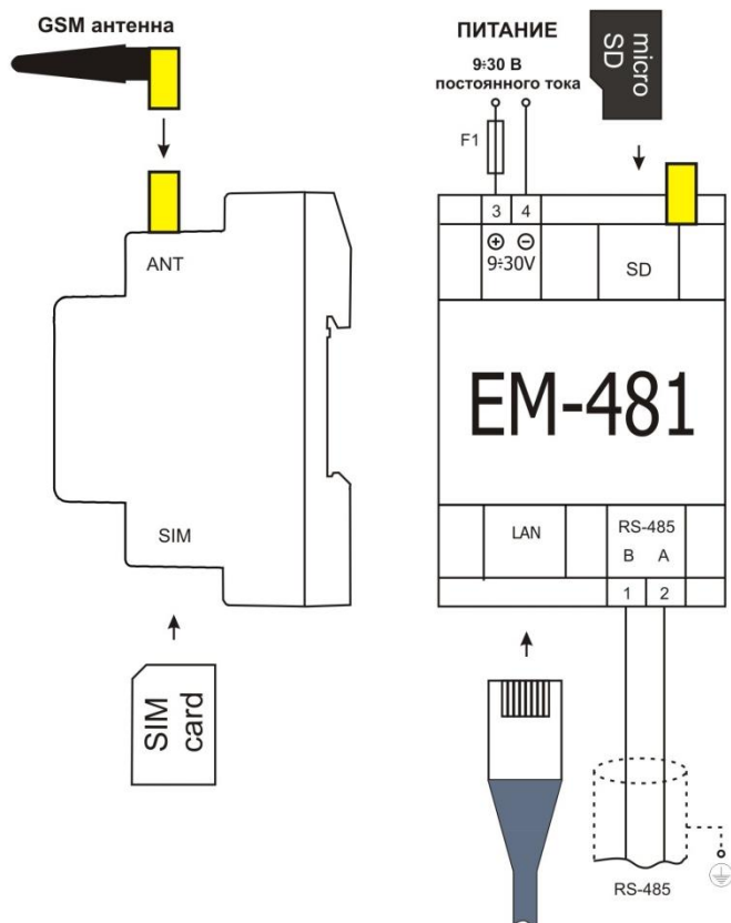
Рисунок 5.1 – Схема подключения изделия
